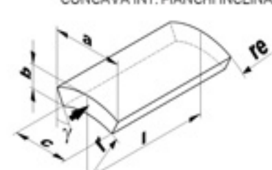
SO SETTORE A SEZIONE TRAPEZIO ISOSCELE
