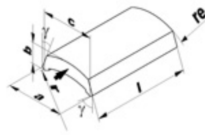
SG SETTORE A SEZIONE TRAPEZOIDALE CONVESSA EST. CONCAVA INT. SMUSSATA
