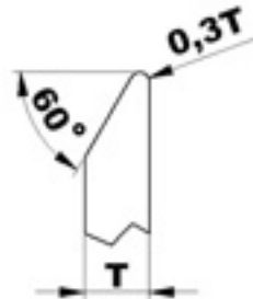
D MOLA A DISCO PROFILATA
