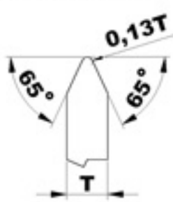
G MOLA A DISCO PROFILATA
