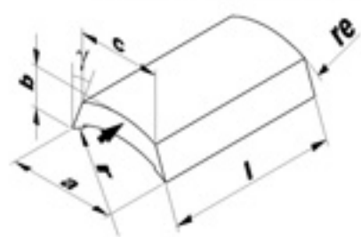
SE SETTORE A SEZIONE TRAPEZOIDALE CONVESSA EST. CONCAVA INT. SCARICATA
