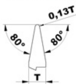
H MOLA A DISCO PROFILATA
