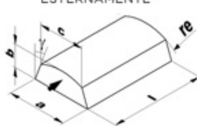
SE SETTORE A SEZIONE TRAPEZOIDALE CONVESSA EST. CONCAVA INT. SCARICATA
